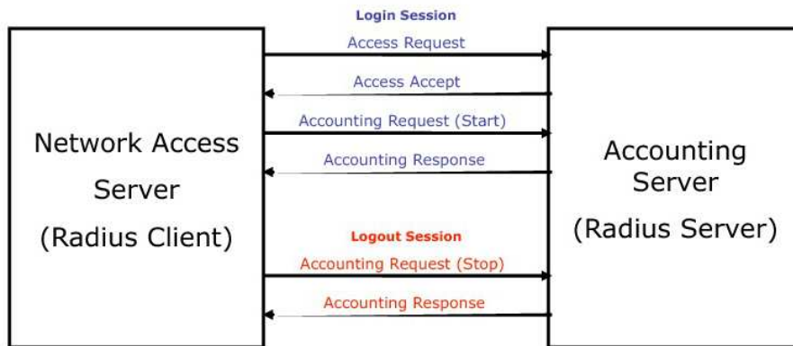
Figura 22: Il protocollo RADIUS
