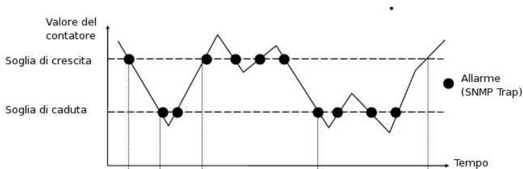
Figura 7: RMON: allarmi
