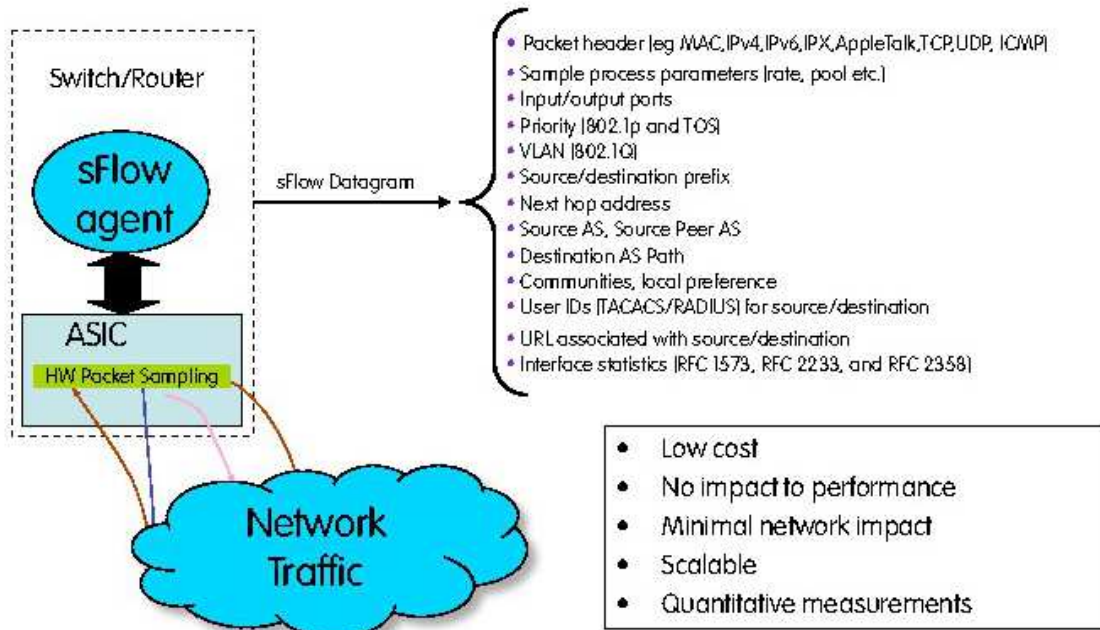
Figura 20: sFlow: sommario
