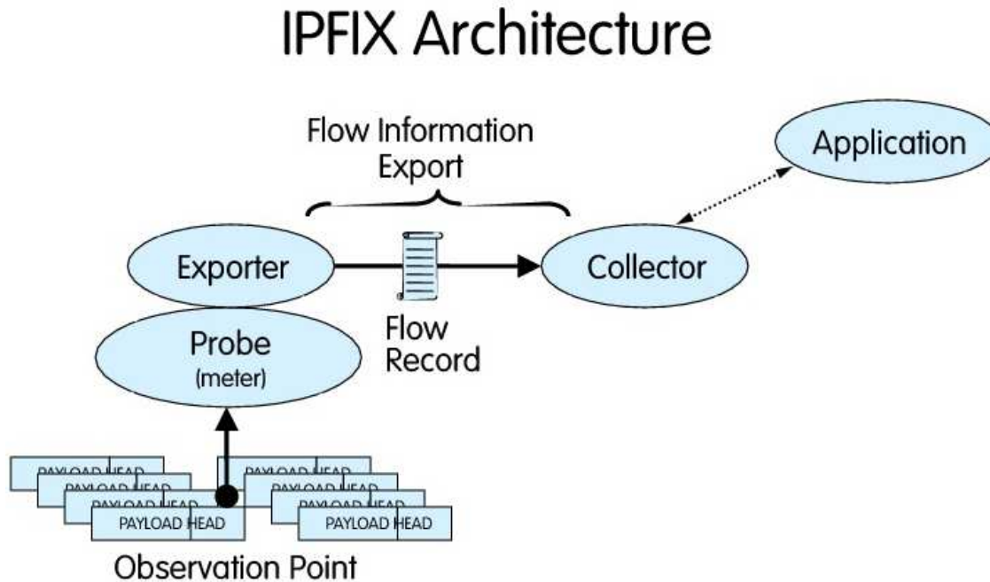
Figura 19: Architettura di IPFIX
