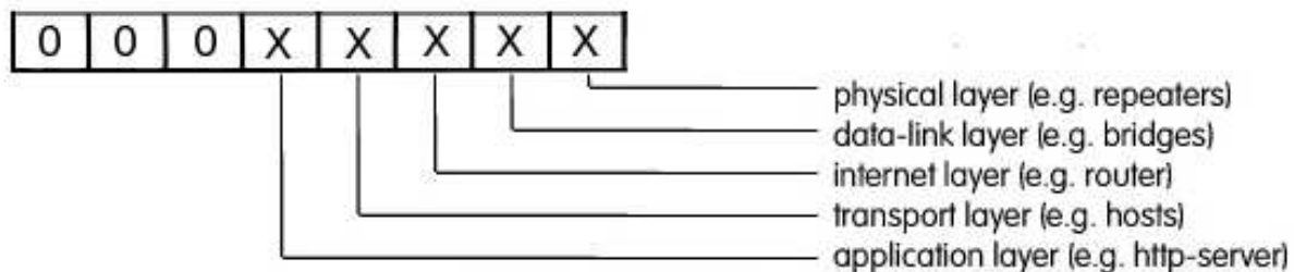
Figura 2: MIB II: gruppo "system", variabile sysService
