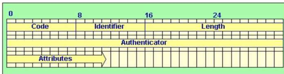
Figura 23: Messaggi del protocollo RADIUS
